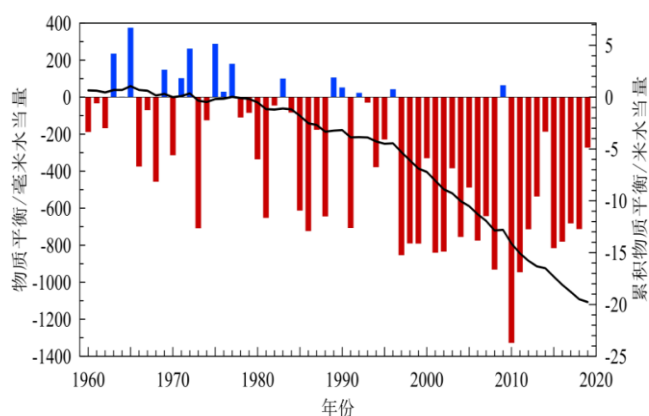
1960~2019年天山烏魯木齊河源1號冰川物質平衡（直條圖）和累積物質平衡（曲線，相對於1970年）變化
