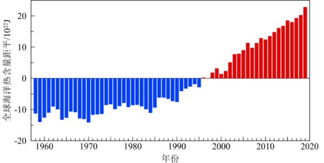
1958～2019年全球海洋熱含量（上層2000米）距平變化
