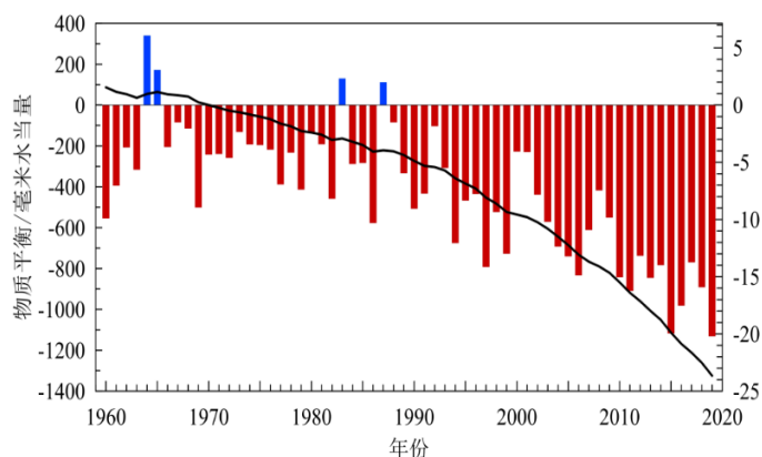
1960~2019年全球參照冰川平均物質平衡（直條圖）和累積物質平衡（曲線，相對於1970年）變化
