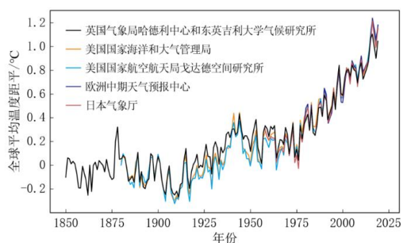
1850～2019年全球平均溫度距平（相對於1850～1900年平均值）
