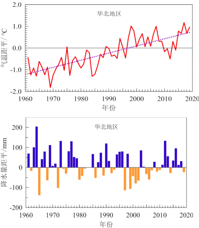
1961～2019年中國八大區域年平均氣溫距平和年降水量距平變化（點線為線性變化趨勢線）
